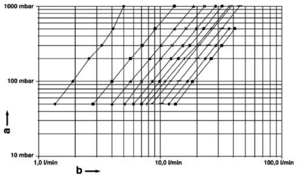
Bild 2 Druckverlustdiagramm für Regulierventil am Rücklauf a - Druckverlust [mbar] b - Volumenstrom [l/min]
