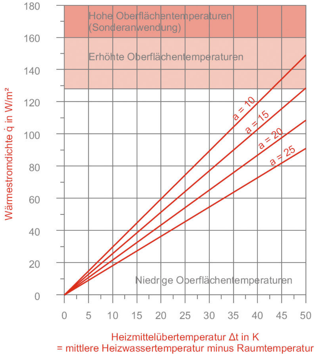
Diagramm 12 Oberbelag R_s = 0,15 \text{ m}^2\text{K/W}
