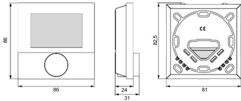
Abmessungen (alle Angaben in mm)
