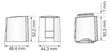
Abmessungen Installationshöhe
