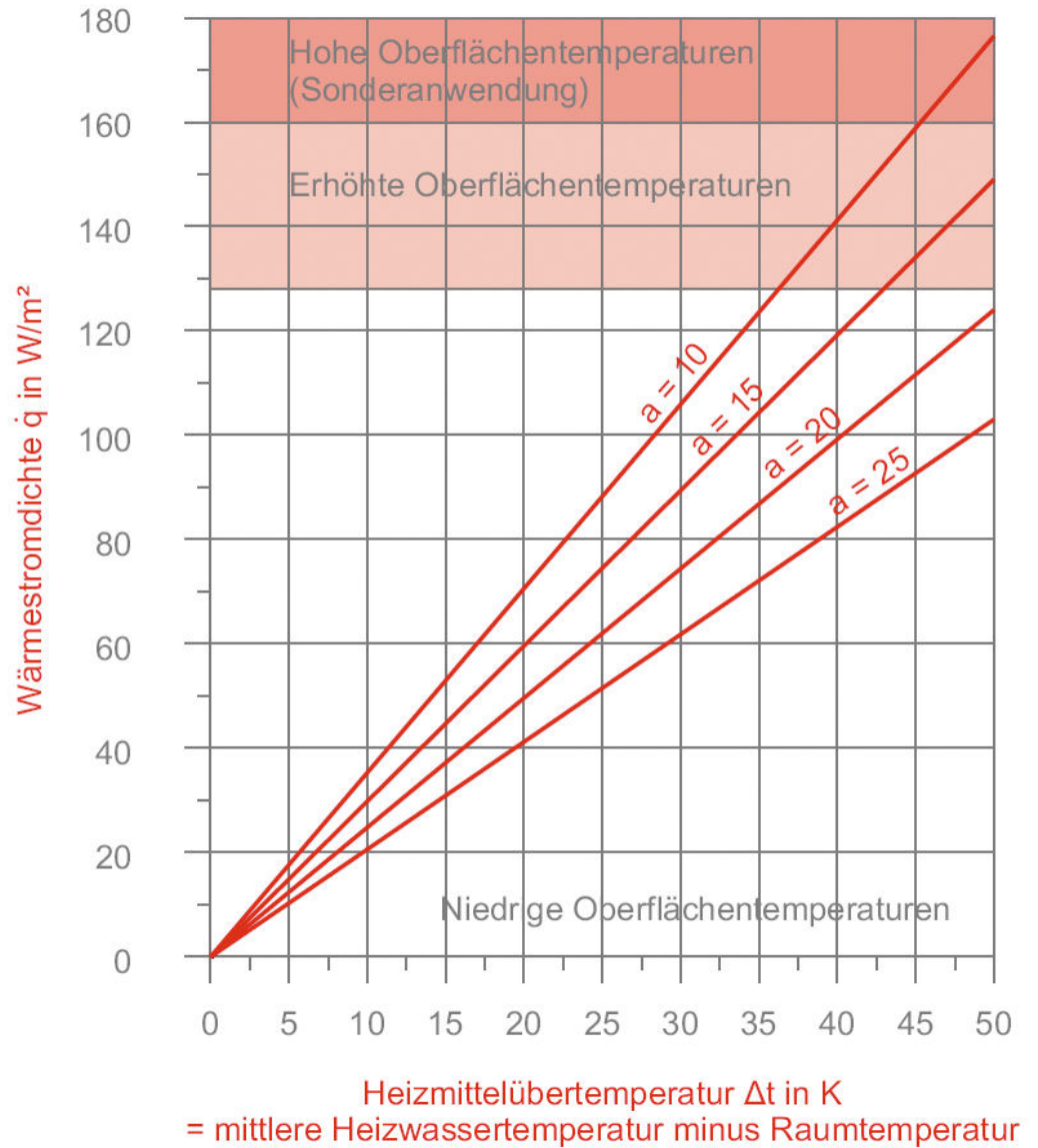
Diagramm 11 Oberbelag R_{\lambda} = 0,10 \text{ m}^2\text{K/W}
