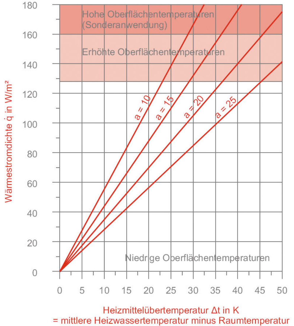
Diagramm 9 Oberbelag R_s = 0,00 \text{ m}^2\text{K/W}
