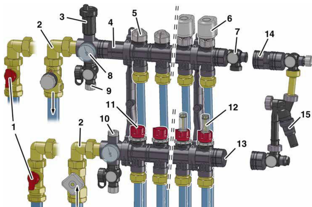
Bild 1: Kunststoffverteiler PA Modular
