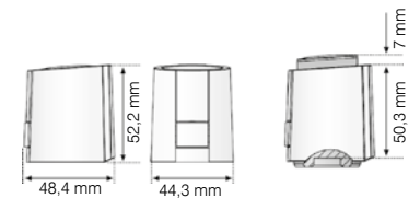
Abmessungen Installationshöhe
